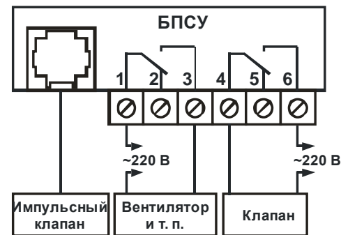
Рисунок 2 – Схема подключения внешнего оборудования к БПСУ
