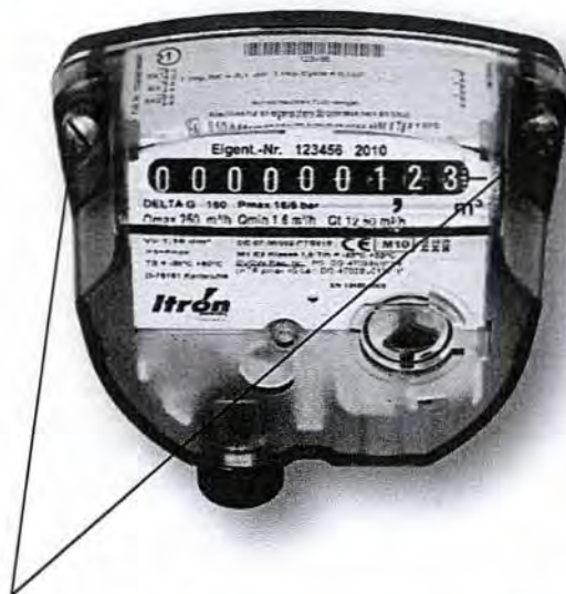
Рисунок 2- Места пломбирования счетчиков газа ротационных Delta Знак поверки наносится на винты крепления крышки отсчетного устройства счетчика.
