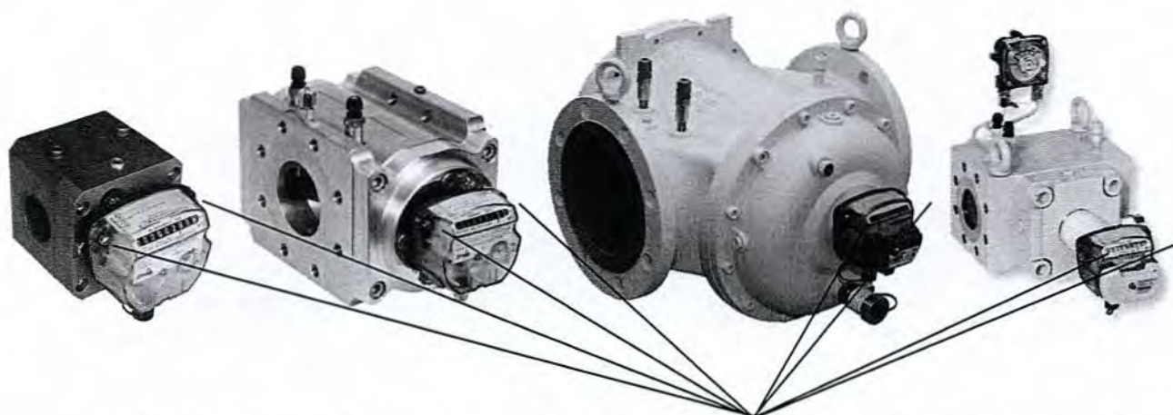
Рисунок 1 - Общий вид счетчиков газа ротационных Delta и мест пломбирования
