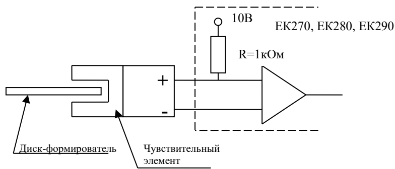
Рисунок 19 – Схема среднечастотного датчика импульсов R300
